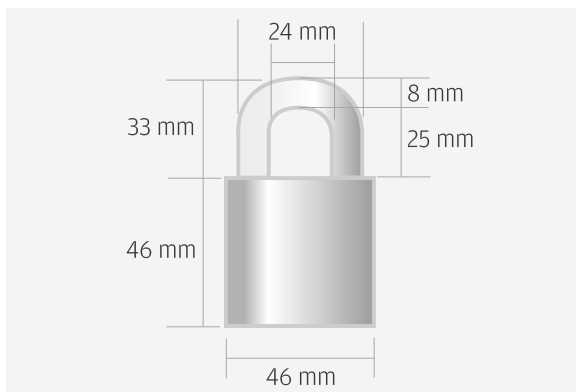
Empfohlene Vorhängeschlösser.
