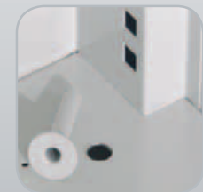
Bodenverankerung
