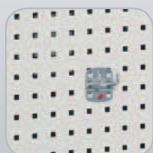
®RasterPlan Lochplatten im Lochabstand 38 mm und Quadratlochung 10 x 10 mm
