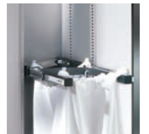
Wäschesackhalterung: In Standardausführung mit vier stabilen Haltehaken (Bild Mitte) oder als Komforthalterung mit Teleskopauszug zur leichteren Entnahme des Wäschesackes.
