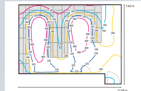
Lichtplanung mit ISO-Linien zur Angabe der Beleuchtungsstärken in Lux an jedem Ort des Raumes
