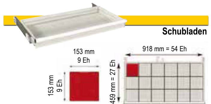
Auszugboden aus Stahlblech
